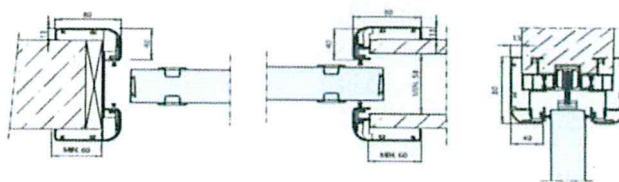
Sezioni apertura scorrevole interno muro.
